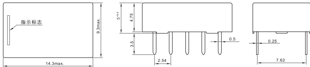
外形尺寸图
