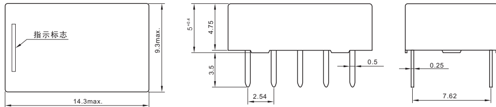
外形尺寸图
