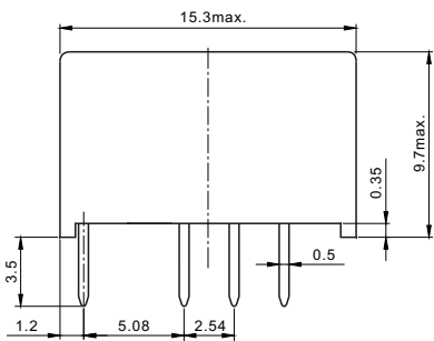
外形尺寸图
