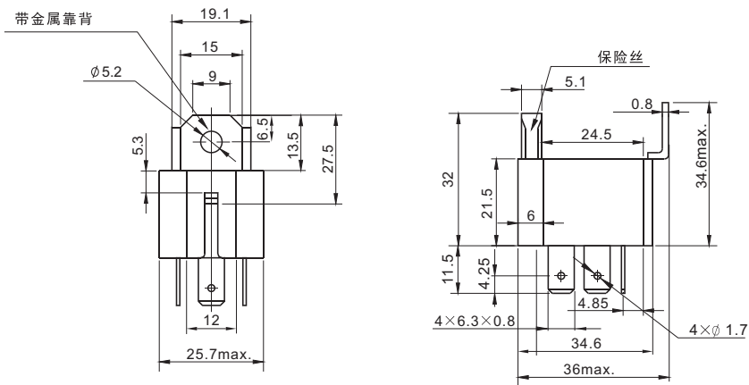
外形尺寸图
