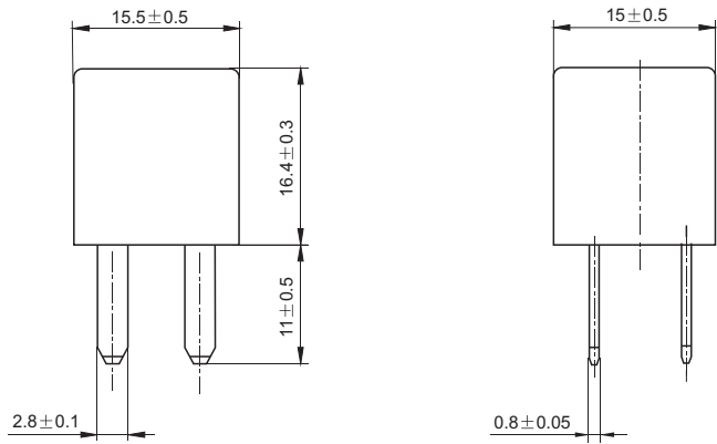
外形尺寸图
