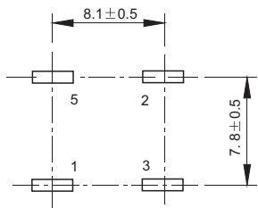
安装尺寸图（底视图）
