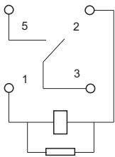
接线图（底视图）
