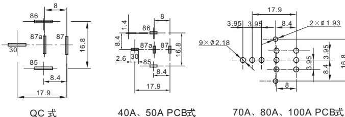
安装尺寸图 (底视图)
