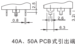
40A、50A PCB式引出端
