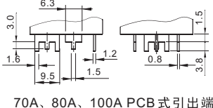
70A、80A、100A PCB式引出端
