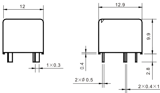
外形尺寸图
