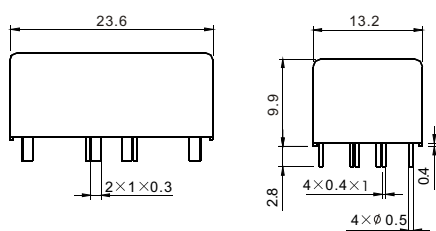
外形尺寸图
