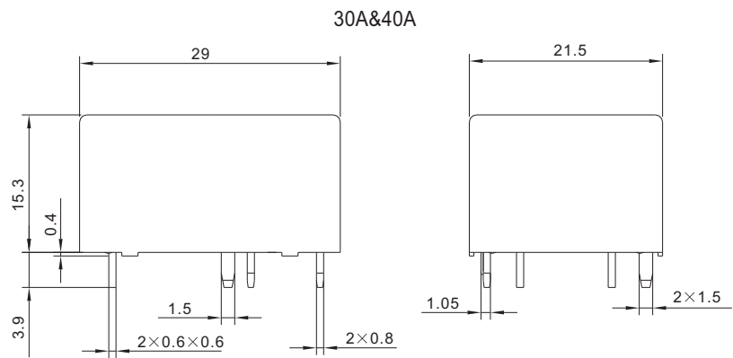
触片脚宽度:标准型 外形尺寸图
