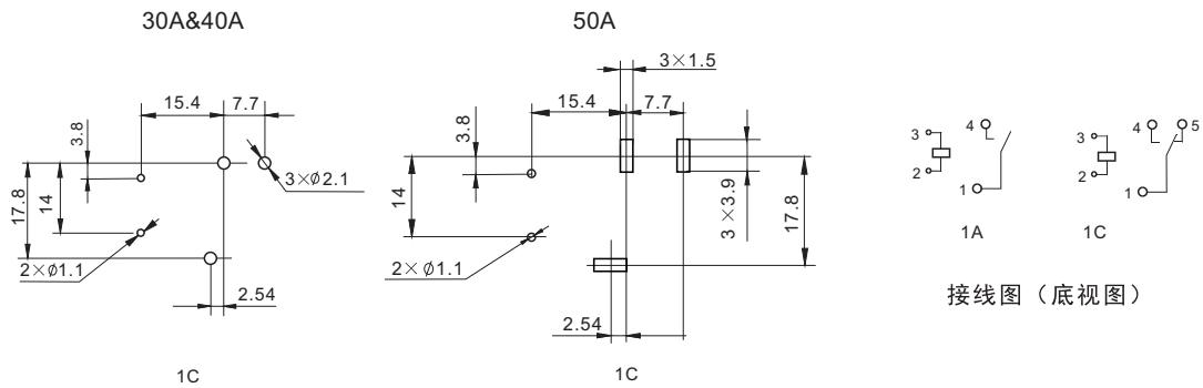
安装尺寸图（底视图）
