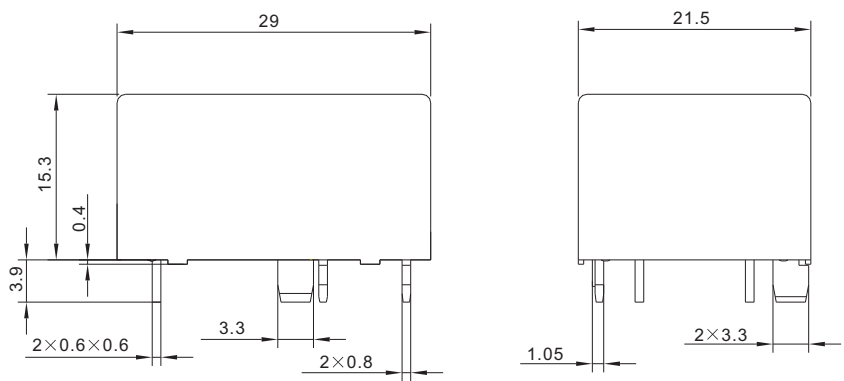
触片脚宽度:3.3mm 外形尺寸图
