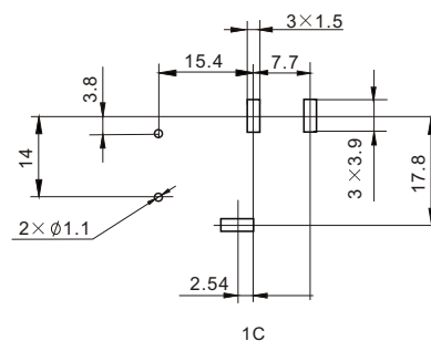
1C 安装尺寸图 (底视图)
