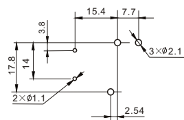
1C 安装尺寸图 (底视图)
