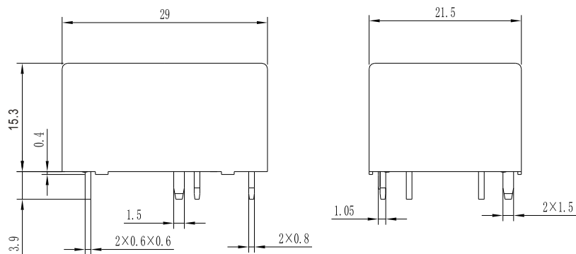
外形尺寸图
