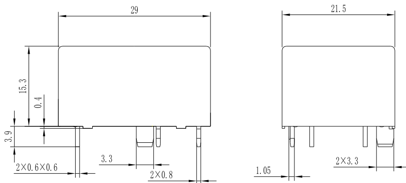
外形尺寸图
