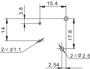
安装尺寸图（底视图）
