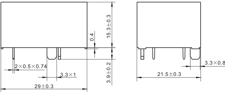
外形尺寸图
