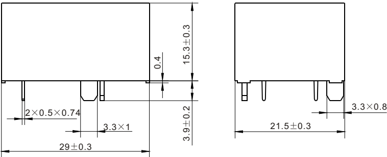
外形尺寸图
