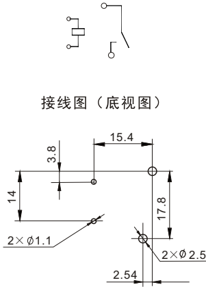
安装尺寸图 (底视图)
