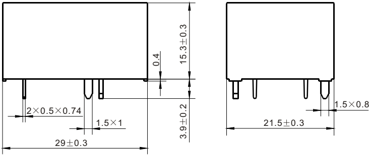
外形尺寸图
