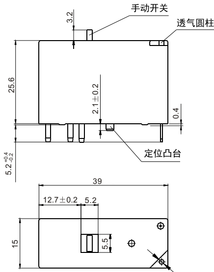
外形尺寸图
