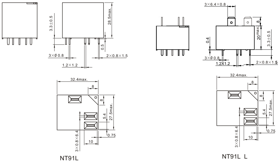
外形尺寸图
