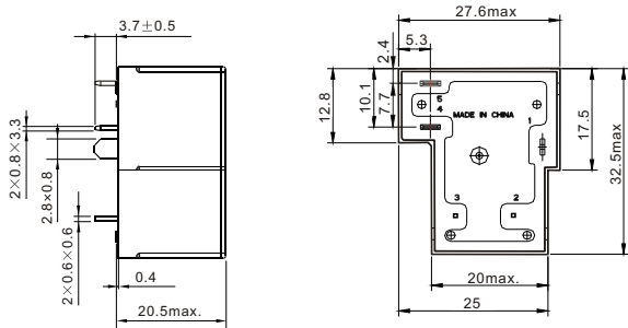
外形尺寸图
