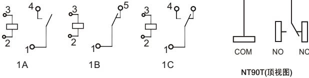
接线图 (底视图)
