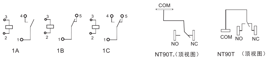
接线图 (底视图)
