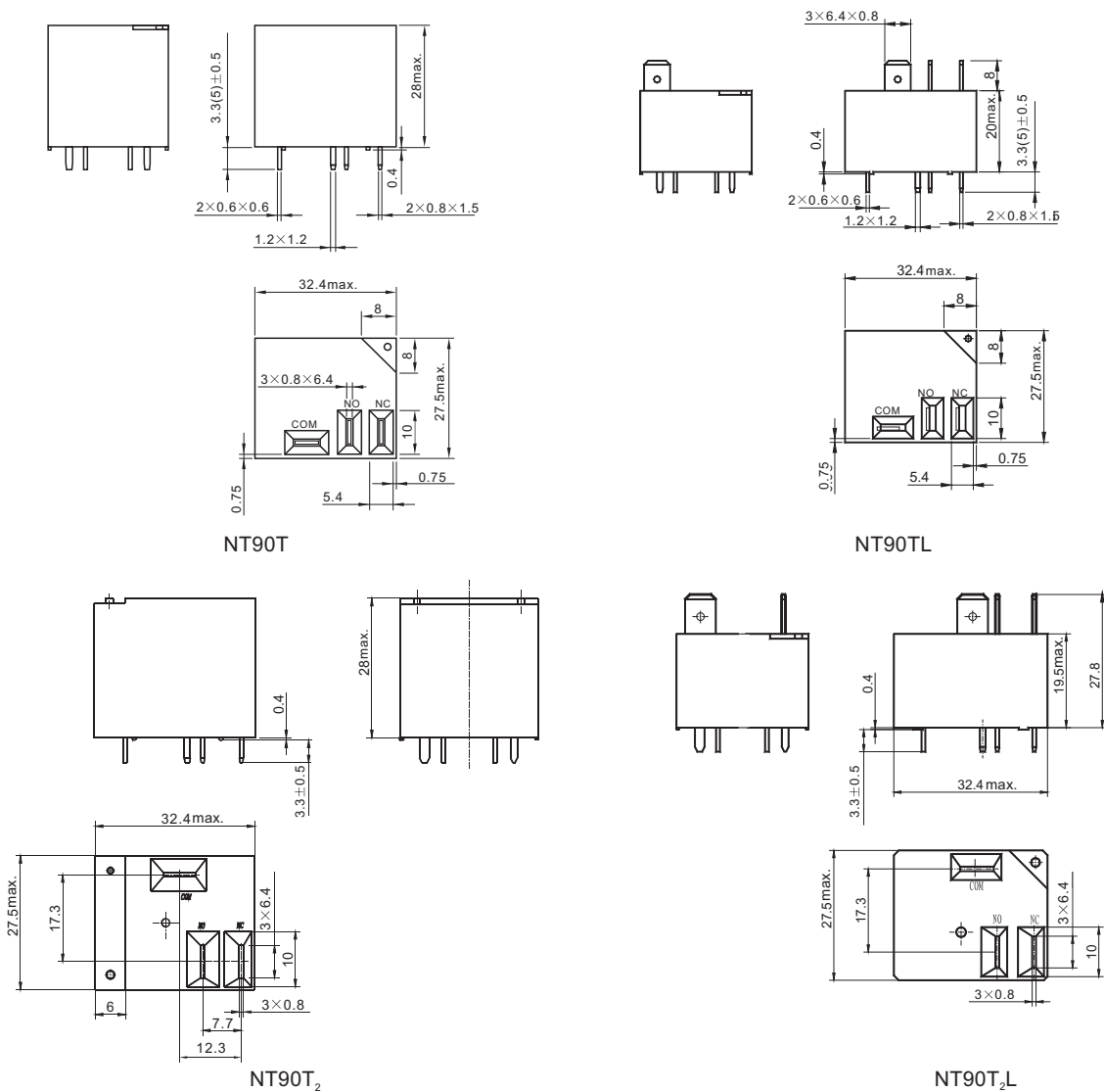
外形尺寸图
