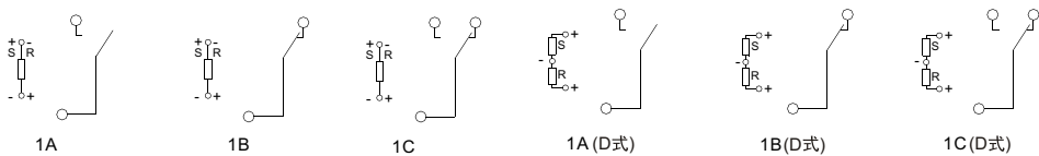
接线图（底视图）
