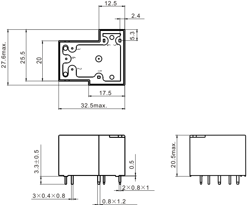
外形尺寸
