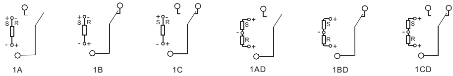
接线图（底视图）
