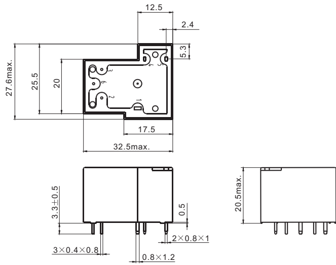
外形尺寸
