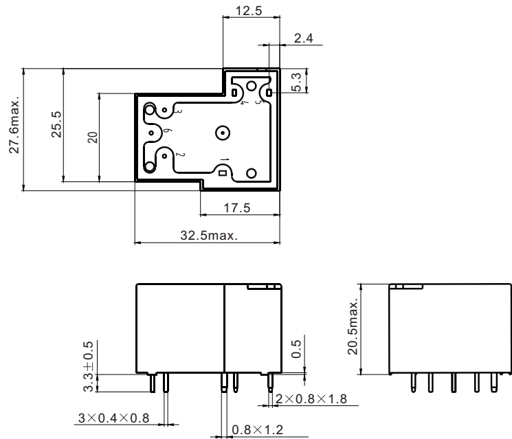
外形尺寸图
