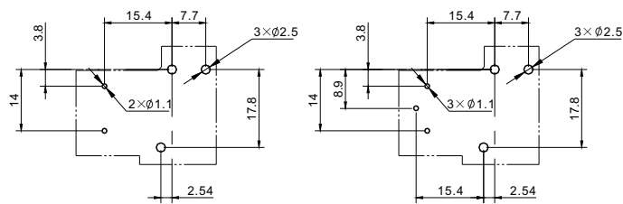
安装尺寸图
