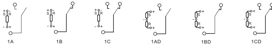
接线图 (底视图)
