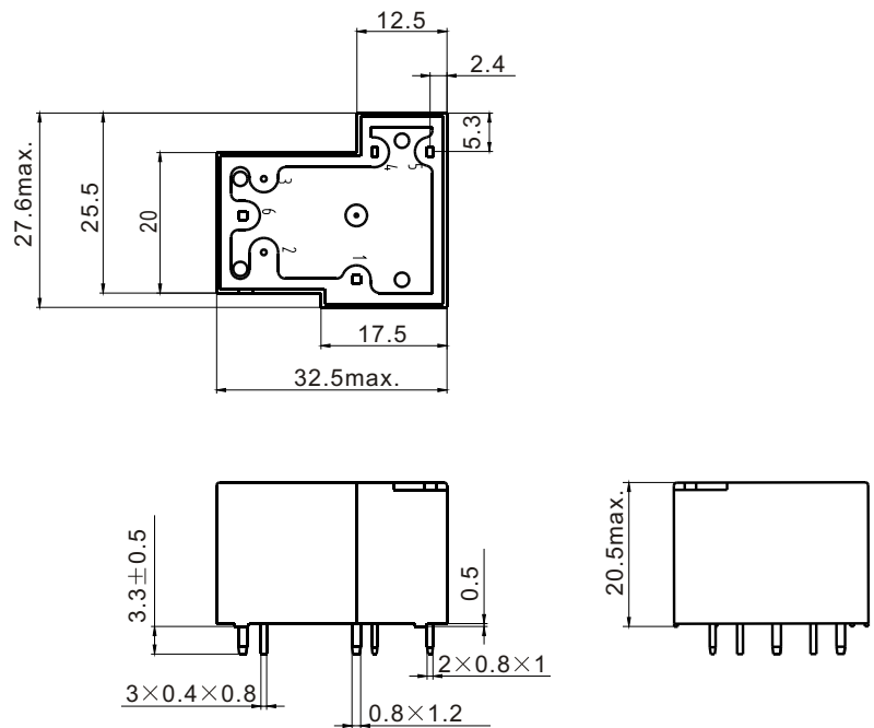
外形尺寸
