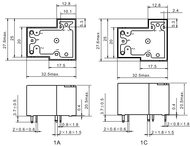
外形尺寸
