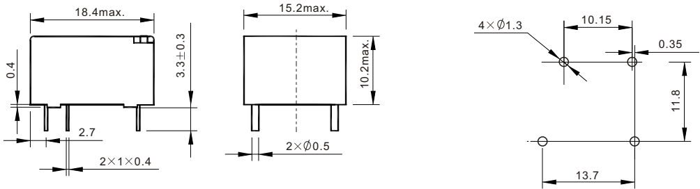
外形尺寸图
