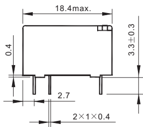
外形尺寸图
