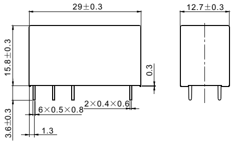
外形尺寸图
