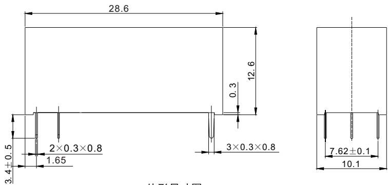
外形尺寸图
