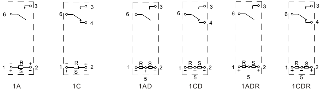
接线图（底视图）
