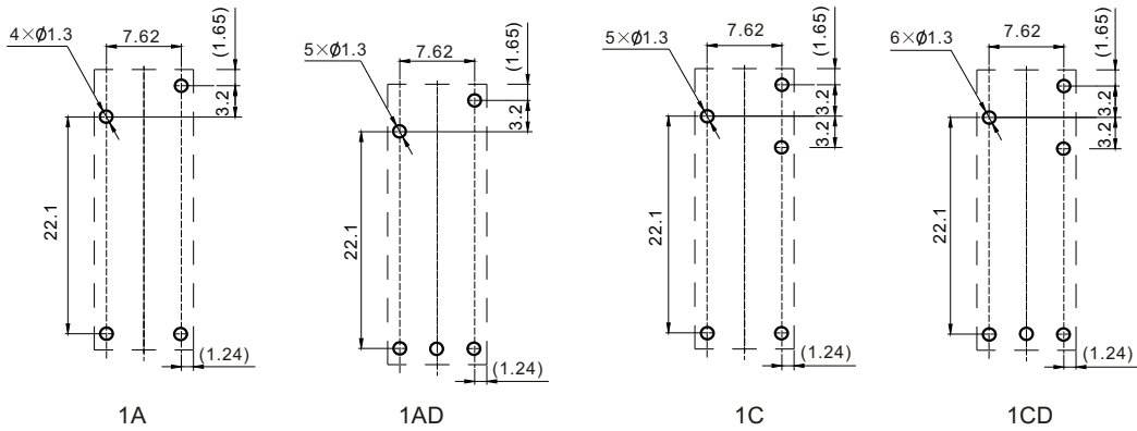
安装尺寸图（底视图）
