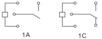
接线图 (底视图)
