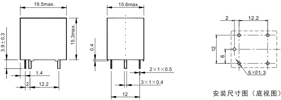
外形尺寸图
