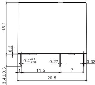
外形尺寸图
