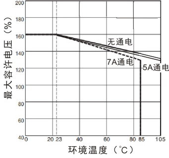
环境温度和最大容许电压
