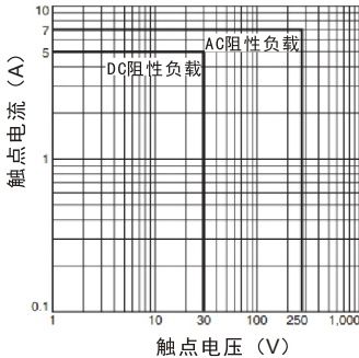
触点切换能力
