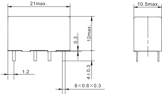
外形尺寸图
