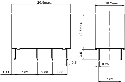
外形尺寸图
