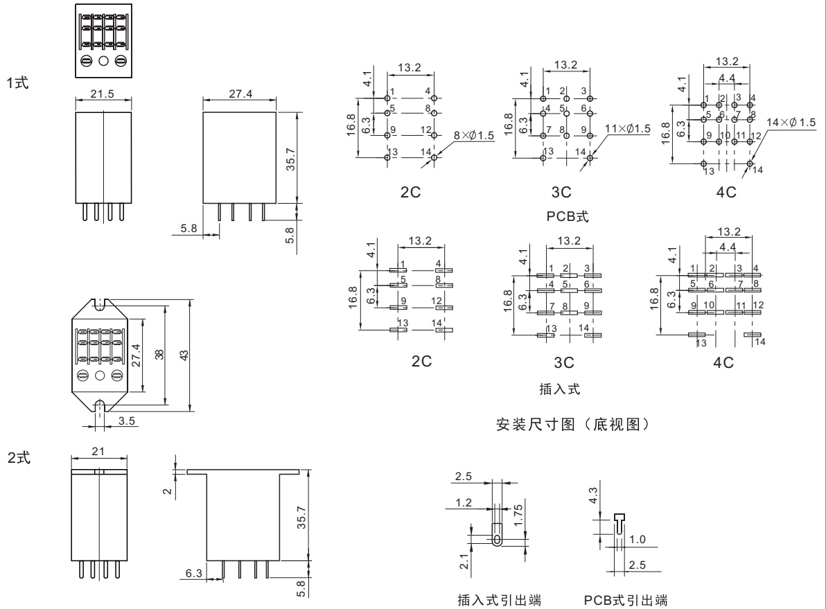
外形尺寸图
