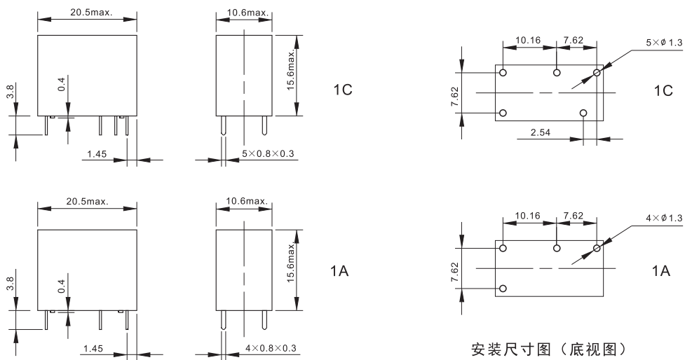
外形尺寸图
