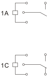
接线图 (底视图)
